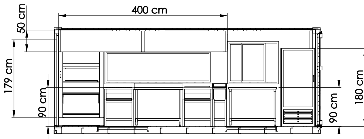
VISTA TRASERA
